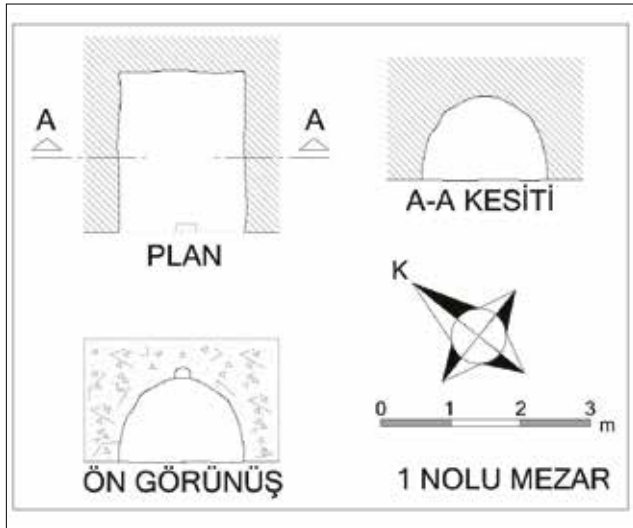
Resim 13: Zile İğdir Köyü Göz Mevkii 1 Nolu Kaya Mezarı Planı / Zile İğdir Village Göz Location, The Plan of Rock Tomb 1
