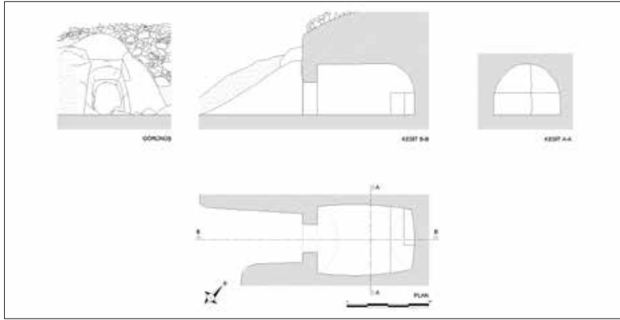
Fotoğraf 3: Boğazkesen Kaya Mezarı, Görünüş, Kesit ve Plan Çizimi / Boğazkesen Rock Tomb, View, Profile and Plan Drawing
