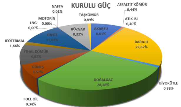
Şekil 1. Türkiye 2019 yılı kaynak bazlı kurulu güç dağılımı (TEİAŞ, 2019) (Elektrik port, 2020)
