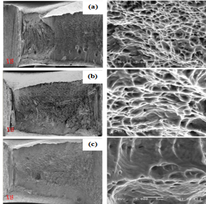
Şekil 12. Çentik darbe deney numunelerinin kırılma yüzeyi SEM görüntüleri (a) 3500W-90cm/min, (b) 3500W-180cm/min, (c) 3500W-270cm/min (The fracture surface of Charpy V-Notch test samples (a) 3500W-90cm/min, (b) 3500W-180cm/min, (c) 3500W-270cm/min).
