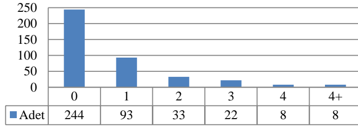
Şekil 21. Traktörlerin motor revizyon sayısına göre dağılımı Figure 21. Distribution of tractors by engine revision number
